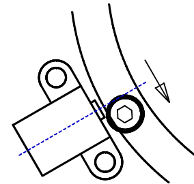
statischer ZZP ca. 6°-8° vOT alle Modelle - Singel- & Twinspark
