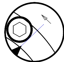
bei ca. 1200 U/min den stehenden Zylinder mit einem Stroboskop im Schauglas abbilden ( bei Racing-Nocken MITTE Schraubenkopf )
