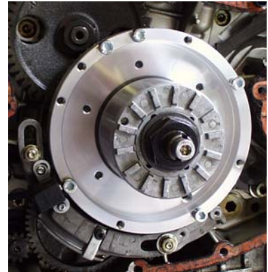
statische Einstellung am Pickup verlassende Schraubenkante -> ca. Mitte Pickup-Kern für den steh. Zylinder (rechts) bei ca. 6°-8° vOT.
