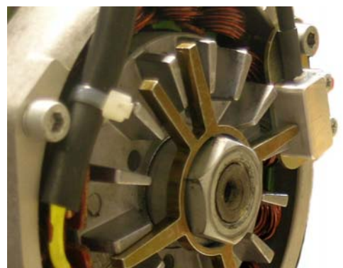
Montage des Hall-Gebers an der Ducati-LiMa mit zwei M5-Schrauben. Der Rotor muss axial mittig zum Alu-Gehäuse mit einem Abstand von 0,4-0,6mm stehen.
