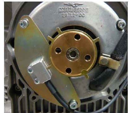
Montage des Hall-Gebers an der SAPRISA-LiMa mit orig. M5 Schrauben und zwei Distanzen Abstand 0,4-0,6mm
