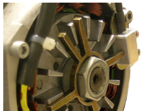
Montage des Hall-Gebers an der Ducati-LiMa mit zwei M5-Schrauben. Der Rotor muss axial mittig zum Alu-Gehäuse mit einem Abstand von 0,6-0,8mm stehen. Vereinzelt müssen durch Fertigungstoleranzen der LiMa die Alurippen abgesägt werden, um den statischen Zündzeitpunkt einstellen zu können. Der Hall-Geber darf die LiMa-Drähte nicht berühren !
