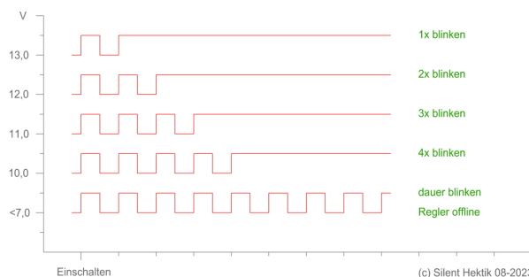
Batterie-Prüfung beim Einschalten mit Blinkcode
